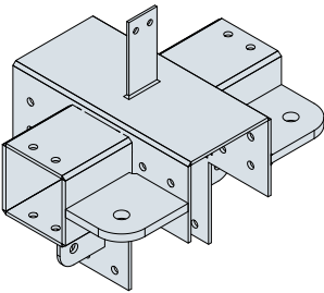
Conexão soldada mecanicamente
