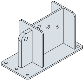
Conexão de contraventamento
